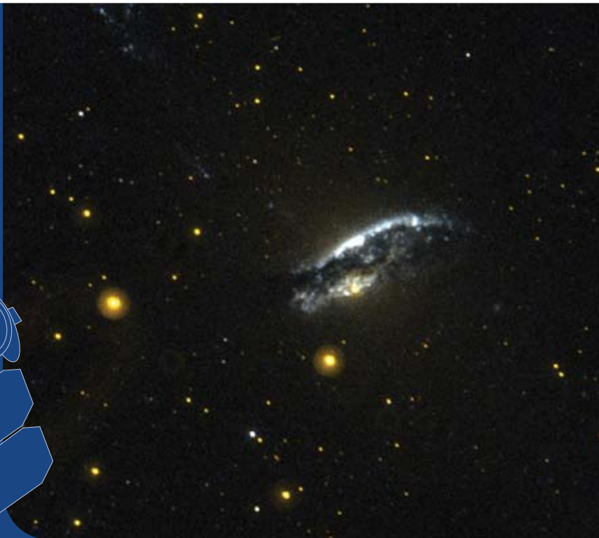
Centaurus A
